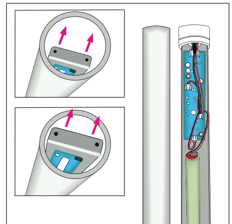
Entfernen Sie die Endkappe und schieben Sie die Schiene vorsichtig heraus, ohne das sich die Innenfolie verschiebt.
