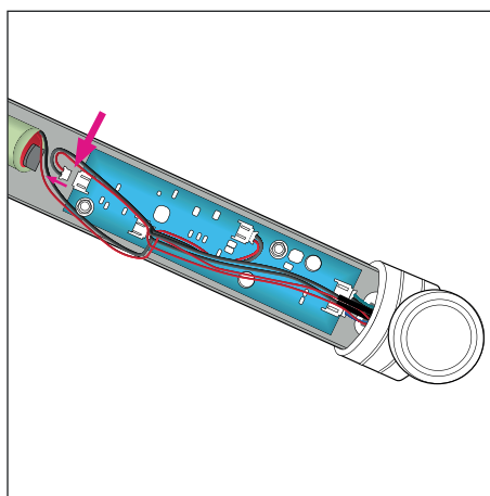
Akkukabel aus der Platine entfernen.
