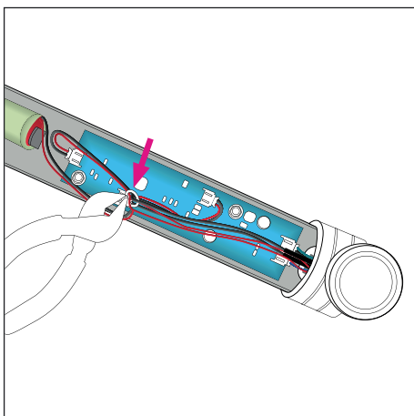
Kabelbinder vorsichtig mit dem Feinmechaniker-Seitenschneider durchtrennen.
