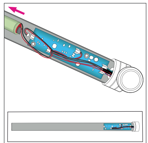
Akku vorsichtig von der Metallschiene lösen. Schiene dabei nicht durchbiegen.
